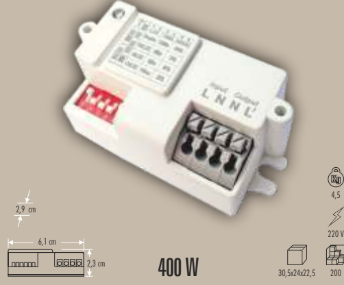
CT-9189 FOTOSEL
